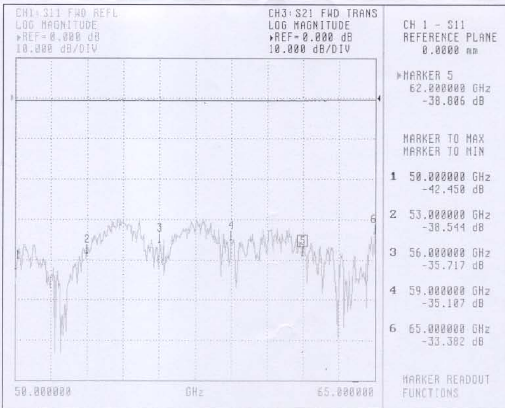
Figure1. H-Plane 90° Bend S11(50-65GHz)
