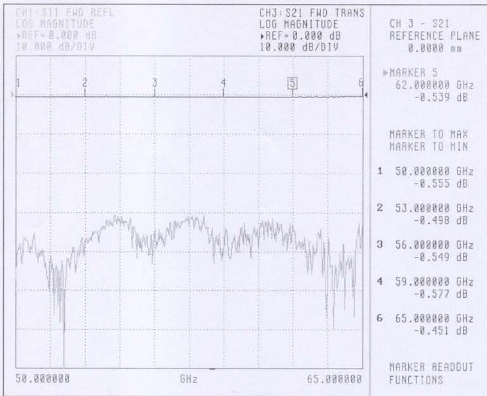
Figure1. H-Plane 90° Bend S21(50-65GHz)
