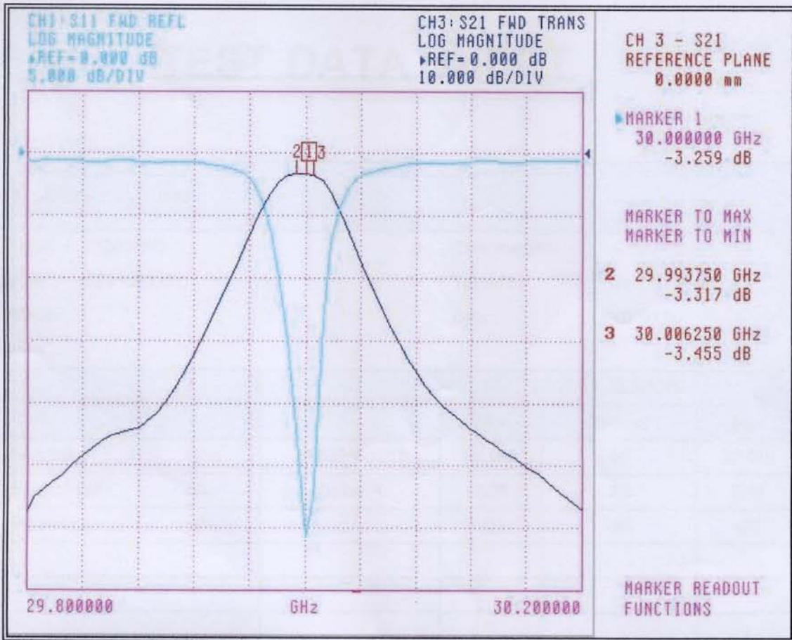
Figure1. S21
